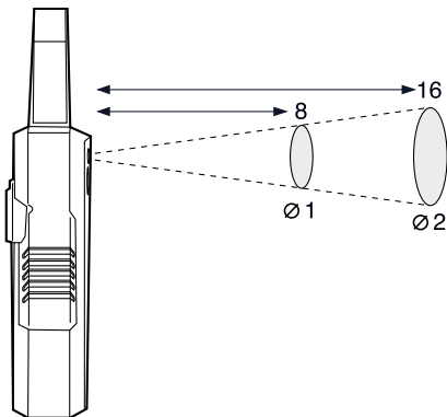
그림 5.2 IR 표적거리비
