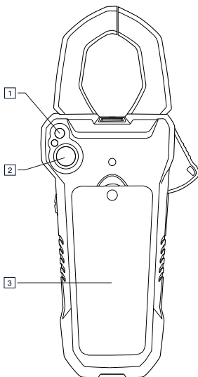
그림 4.2 후면
