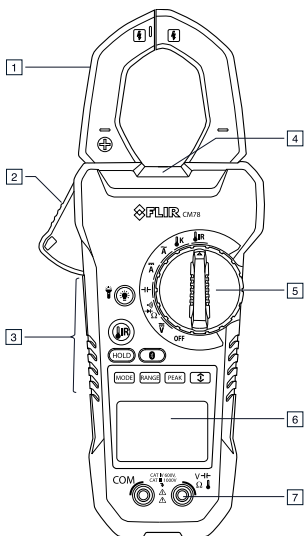
그림 4.1 앞면
